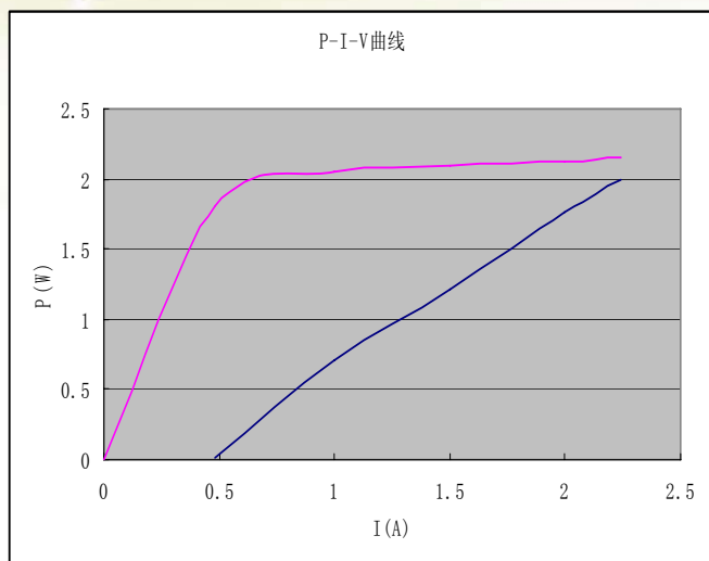
P-I-V 曲线
