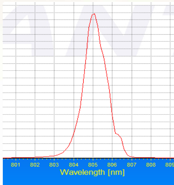
光谱曲线
